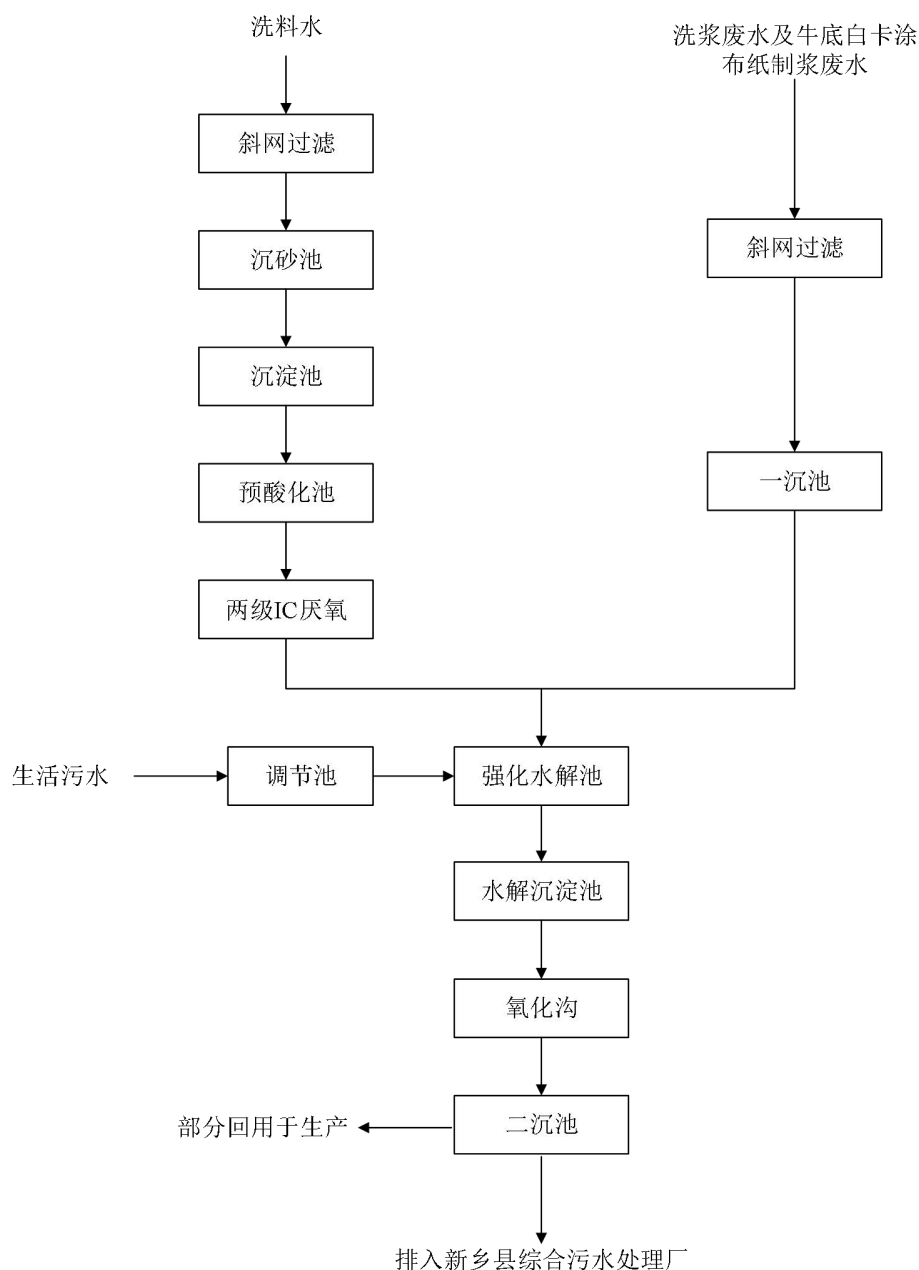
图 6.3-2 兴泰纸业现有综合废水处理工艺流程图
