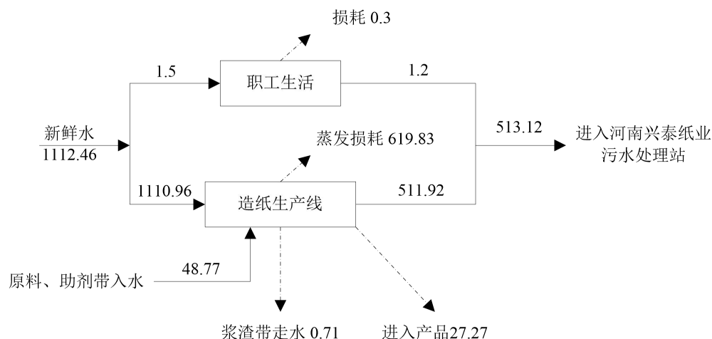
图 3.1-6 本次拟建工程全厂水平衡图（单位：t/d）
