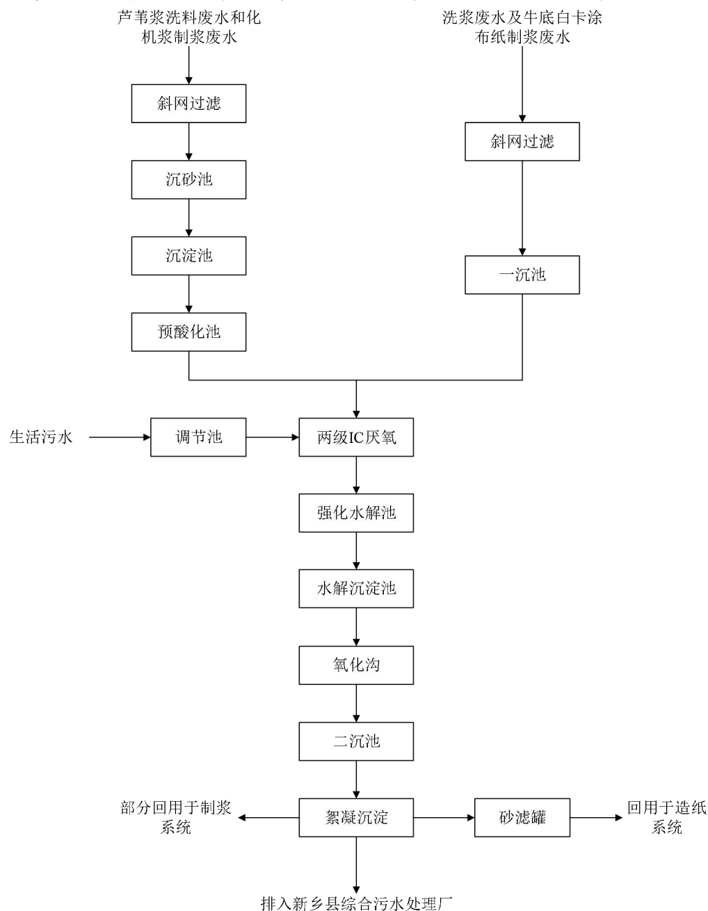
图 6.3-3 兴泰纸业改造后综合废水处理工艺流程图
