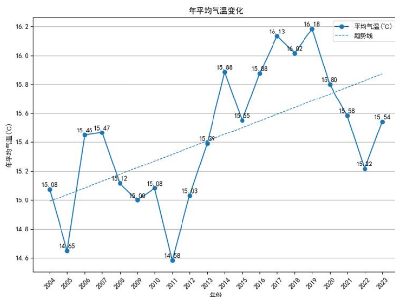
图 5.1-6 新乡年平均气温（单位：℃，虚线为趋势线）
