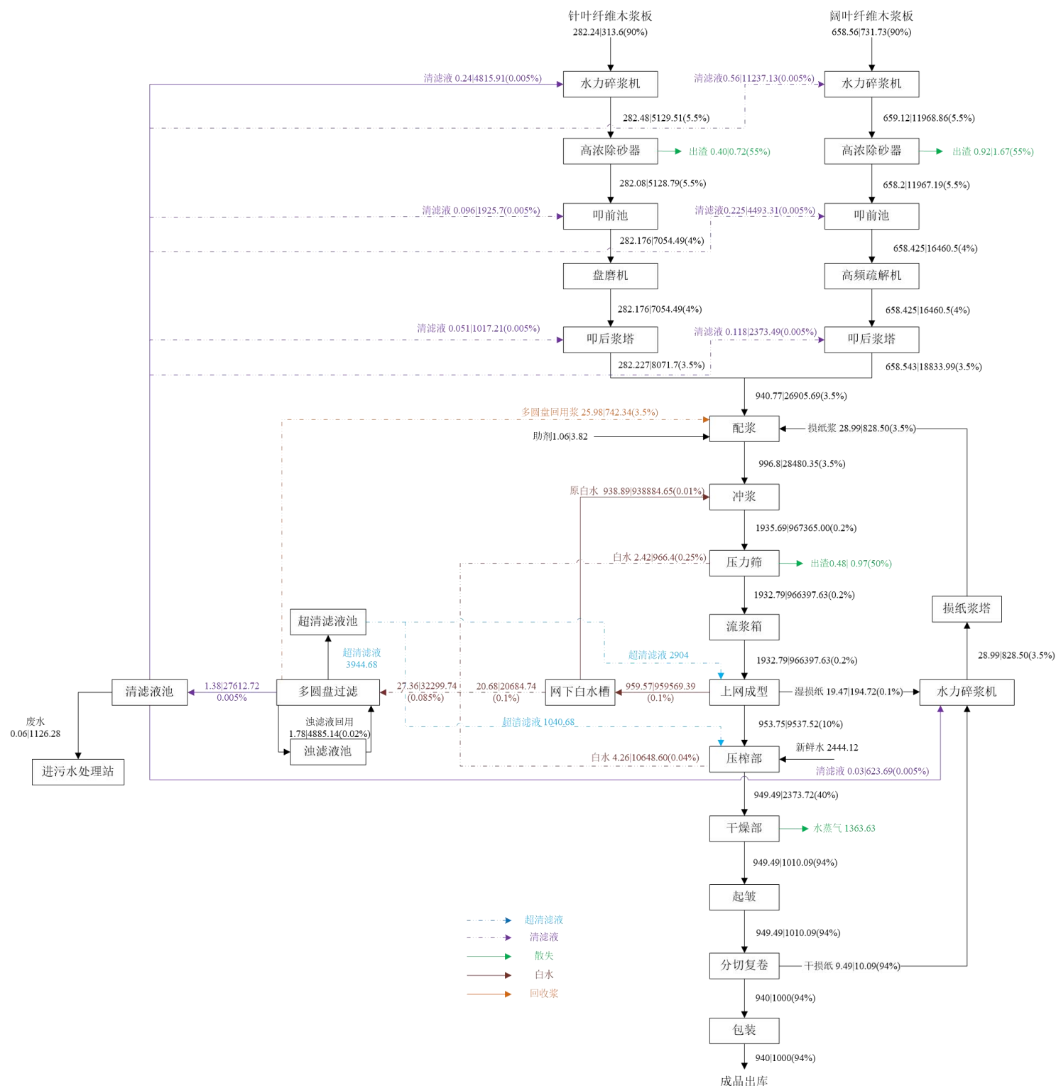
图 3.1-4 本工程生产过程浆水平衡图（绝干浆|浆水(浆浓)单位: kg/t 产品）
